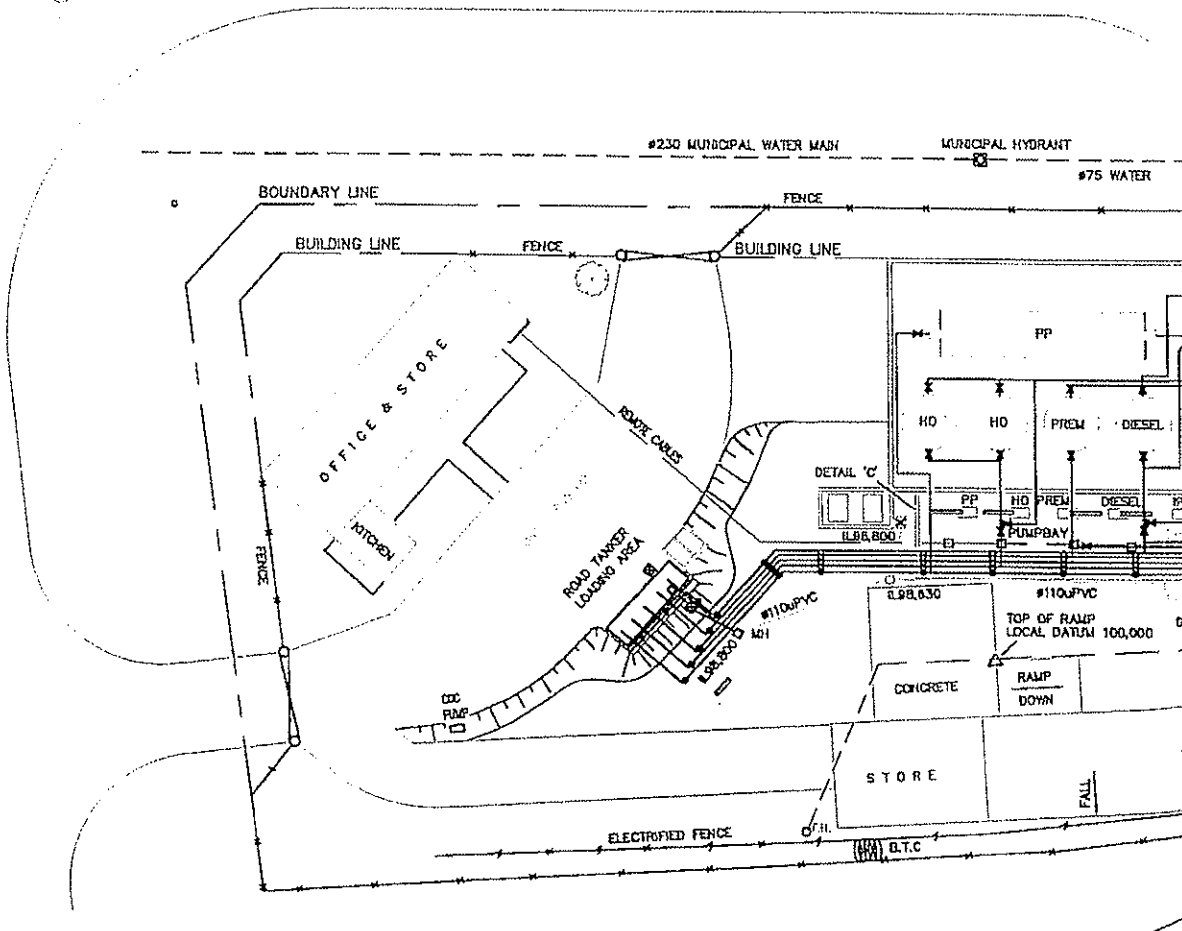
1:200 SITE LAYOUT
